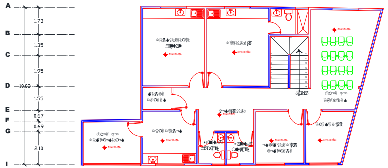
PLANTA ALTA
